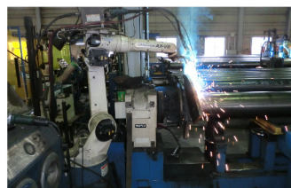
ロボット溶接機
