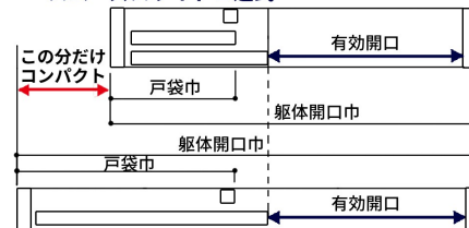
片引戸
