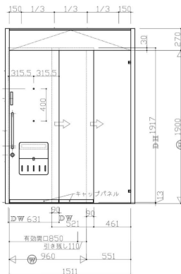
内部側より姿図
