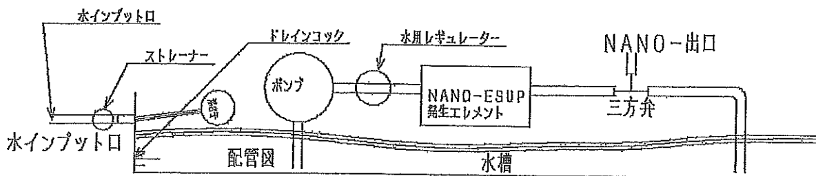
NANO-ESUP 発生装置配管図
