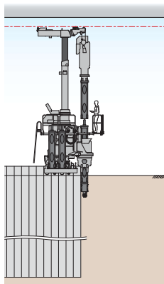
2. 鋼矢板圧入後、 ケーシングを接続
