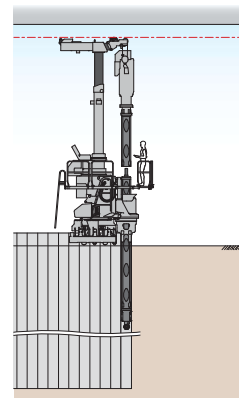
5. 圧入完了後、ケーシ ングを引抜き、ケーシ ング切離し・撤去
