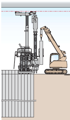
1. 鋼矢板を建て込み
