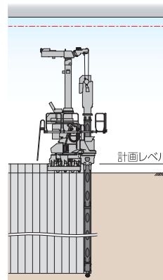
4. 2～3を繰り返し、自走 完了後、鋼矢板を計画 レベルまで圧入
