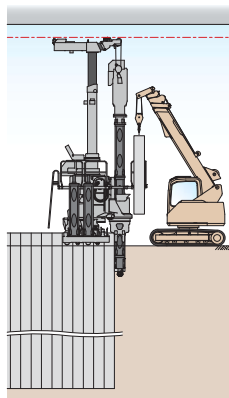
3. 鋼矢板を建て込み、 継溶接
