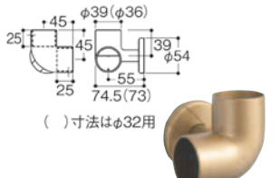
156B-11 縦手すりと横手すりを90°に取付けることができます。
