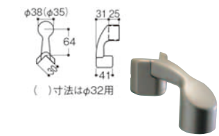
156B-09 柱などの出隅部分に縦手すりを取り付けることができます。
