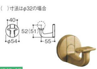
156B-07 墨出しの際、木棒中心位置にブラケットをあわせるだけの施工が簡単です。
