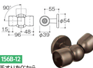
156B-12 手すりを0°から90°の間で自由に曲げて接続することができます。
