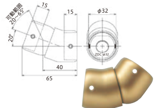
156B-13 20°から65°の間で自由に曲げられます。
