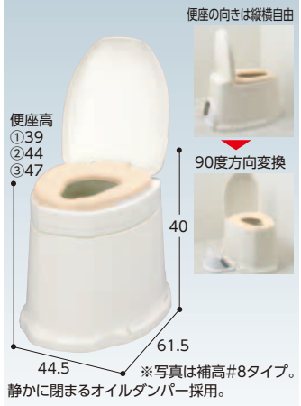
便座の向きは縦横自由 90度方向変換 便座高 ①39 ②44 ③47 40 61.5 44.5 ※写真は補高#8タイプ。 静かに閉まるオイルダンパー採用。 (在) アロン化成
