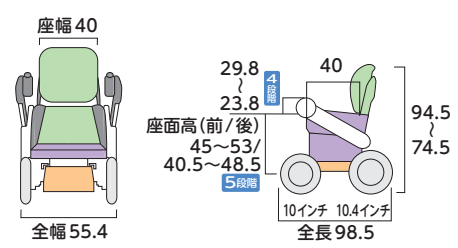
寸法図(単位:cm)
