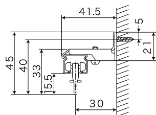
シングルブラケット付
