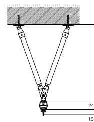
自在吊棒付 (V 吊り)
