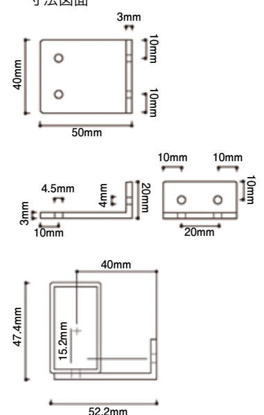
寸法図面
