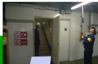
防火ドア動作試験
