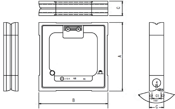
■寸法図 (概略) 単位 : mm
