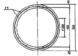
下部側塊
