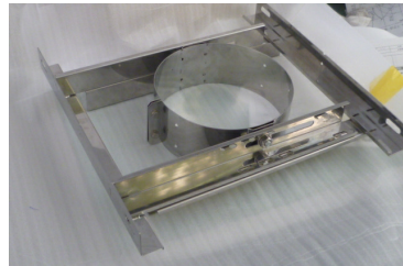
パイプ取付金具 SUS430 t1.5 WDH:300×450×100
