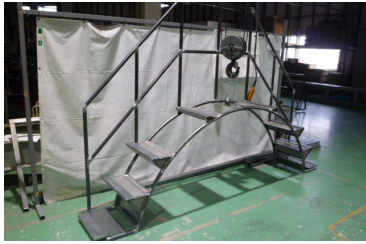
作業用架台 SSパイプ他 WDH:2500×450×2100
