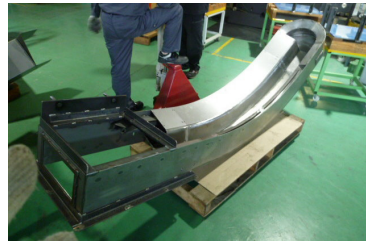
コンベヤフレーム SS t2.3 WHD:350×150×2000
