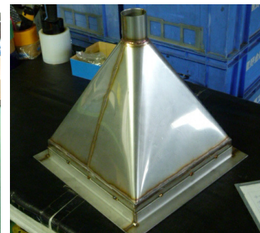
ステンレスホッパー SUS304 t 2.0 WDH:350×350×400
