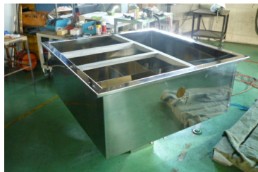
ステンレスホッパー SUS304 t2.0 両研 ※バフあり WDH:1800×1800×800
