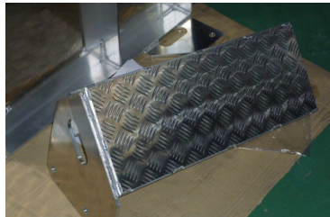
アルミステップ アルミ t6(縞板含む) WDH:450×180×180 アルミ溶接
