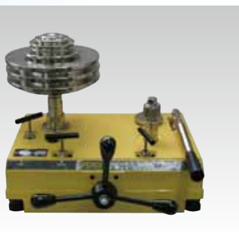
卓上用重錘型圧力計
