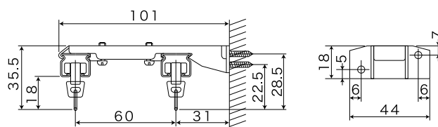
正面付ダブルブラケット T60
