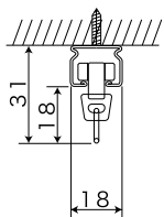
シングル直付
