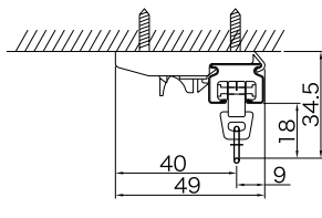
天井付完全ワンタッチ シングルブラケット N
