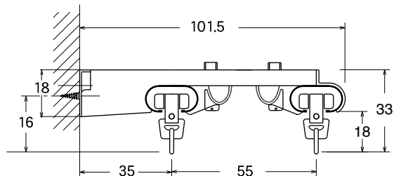
正面付ダブルブラケット T55
