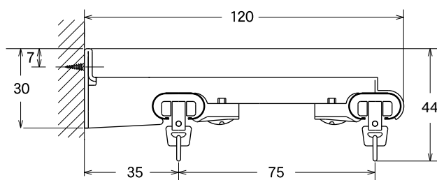
ダブルブラケットロング（公団用）
