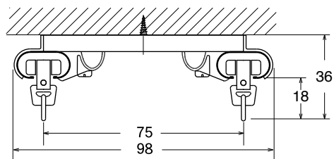
天井付ダブルブラケットロング（公団用）
