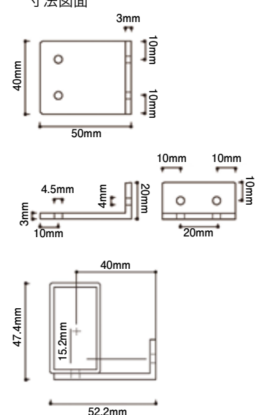
寸法図面
