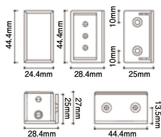
寸法図面
