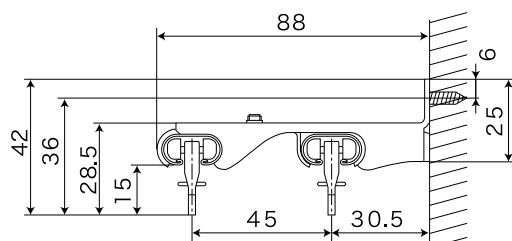
ダブルブラケット付
