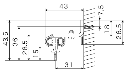
シングルブラケット付
