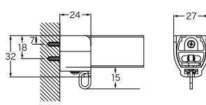
SA サイドブラケット付
