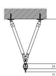
自在吊棒付（V 吊り）
