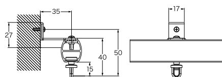
SA 正面 S ブラケット付
