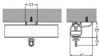
SA 天井 S ブラケット付
