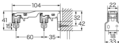
LT ダブルブラケット
