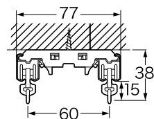
天井付ダブルブラケット
