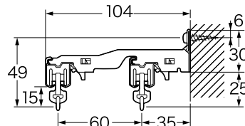
正面付ダブルブラケット
