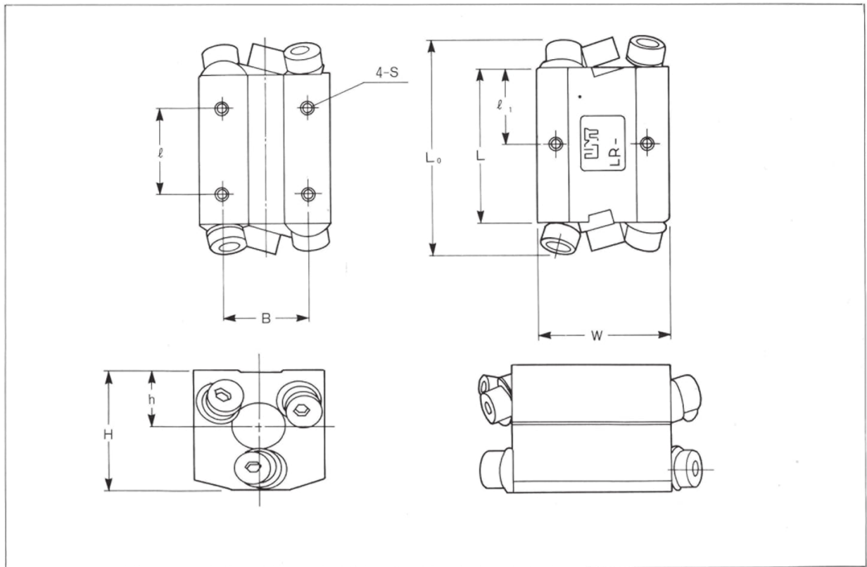
LRシリーズ寸法表
