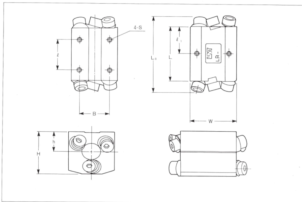
LRシリーズ寸法表
