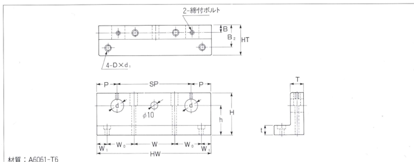
LBEシリーズ寸法表
