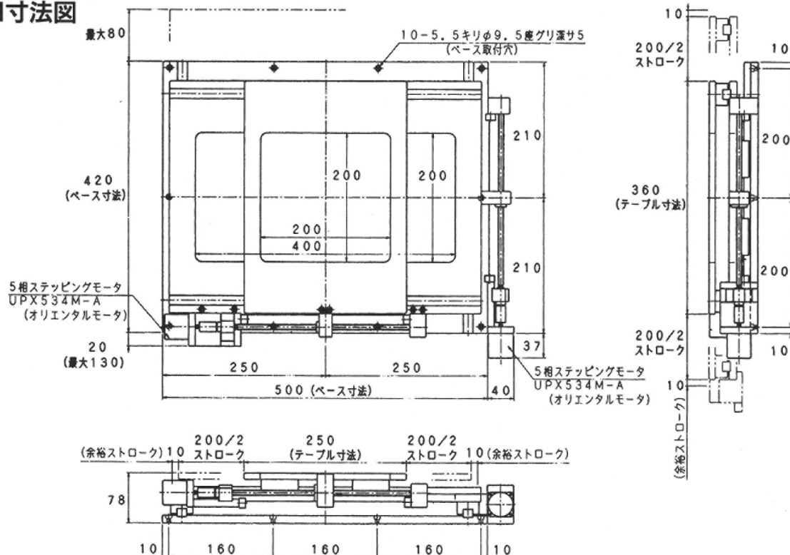
■寸法図
