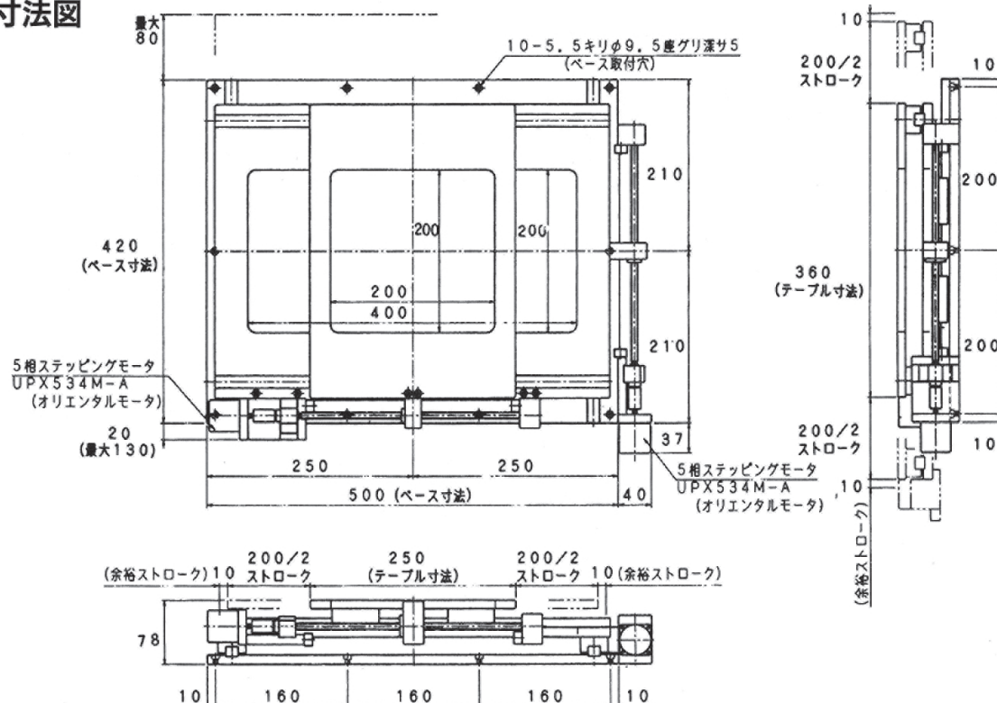
■寸法図
