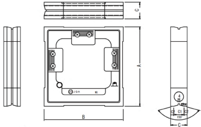
■寸法図 (概略) 単位: mm
